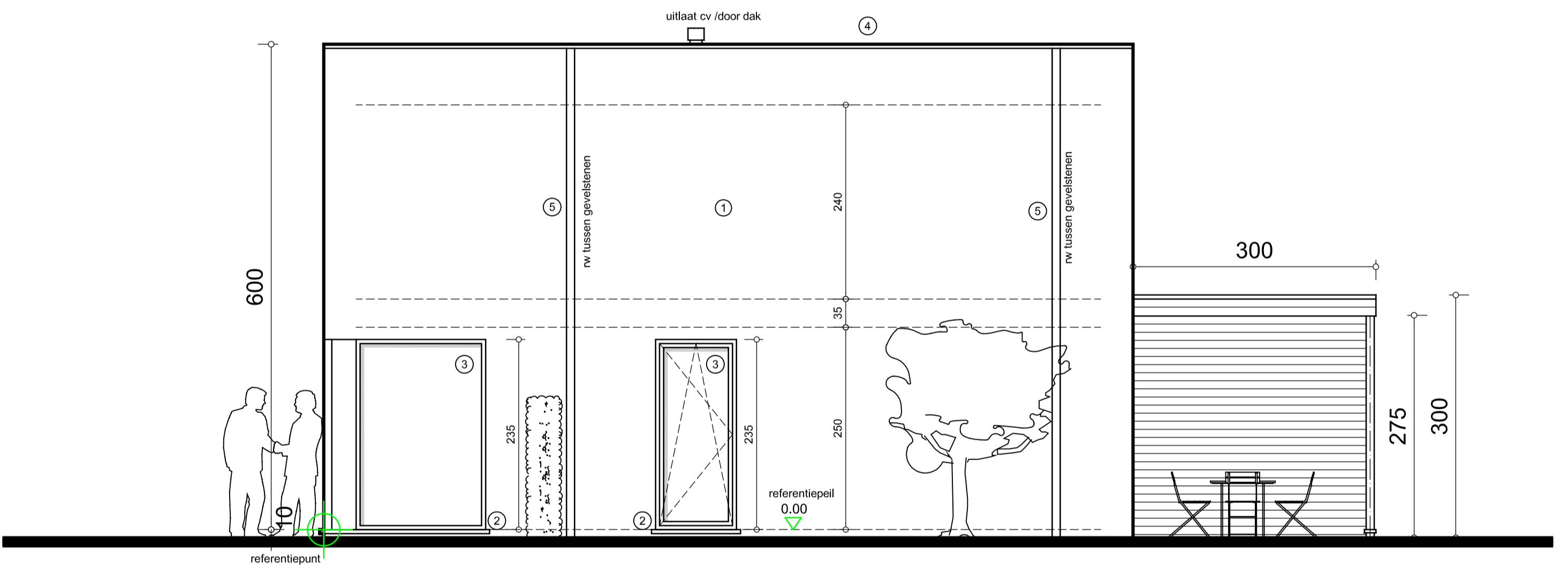
zijgevel rechts / 1:50
